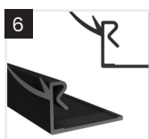
6 Uszczelnienie boczne
