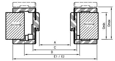
Przekrój poziomy ORB
